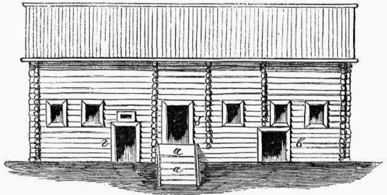
Фасадъ съ боковой стороны.
