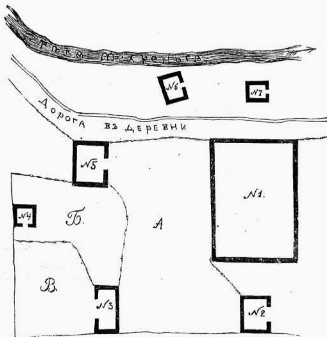
Планъ усадьбы.
